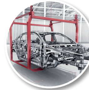
Carrocería y chasis reforzados Chery SMA
